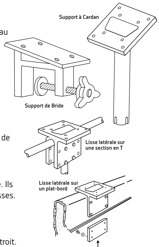
Positions typiques de montage
